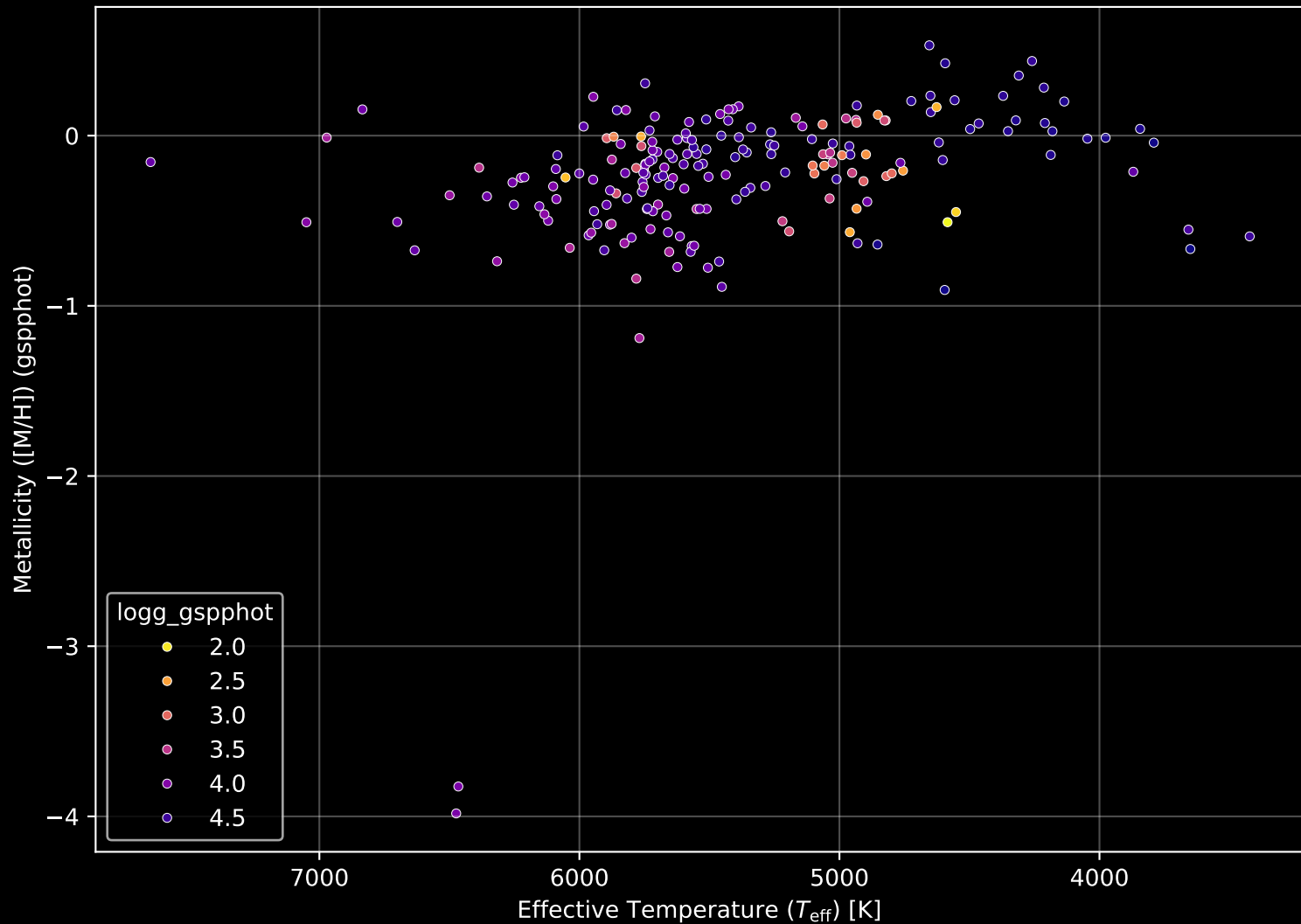
APOGEE DR17 Field: [186-55] Stellar Population Parameters (n= 202)
